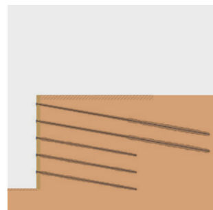
Baugrubensicherung
